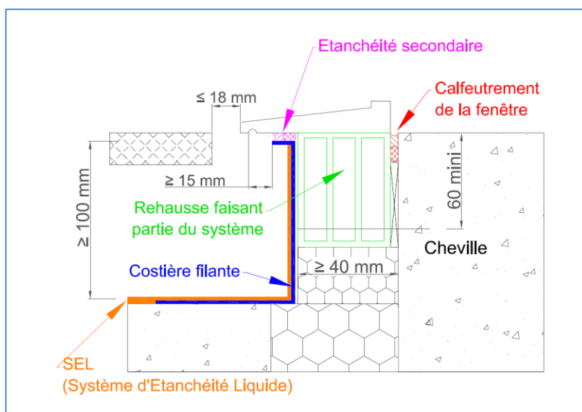
Fig. 7 : Utilisation d'une costière filante pour reconstituer le rejingot
