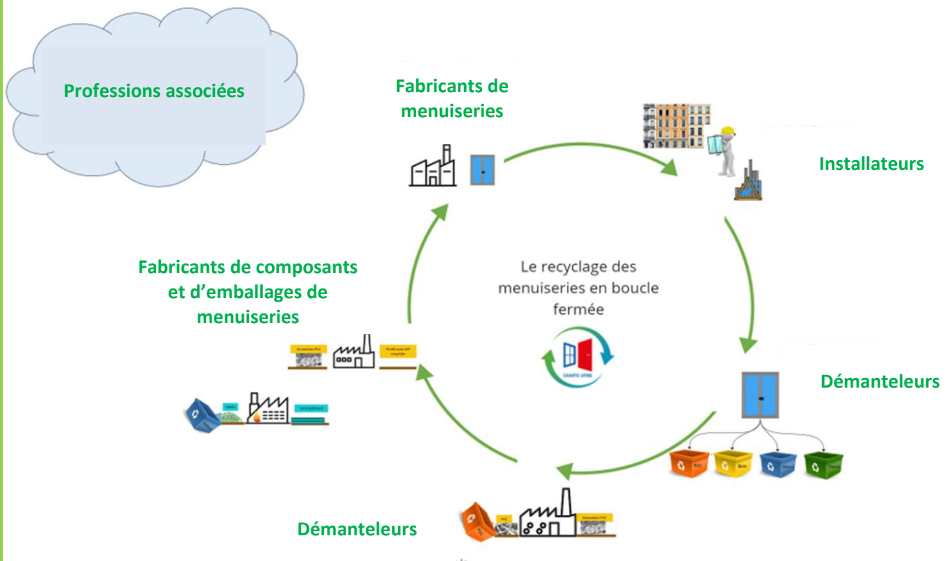
Figure 1: Les acteurs du cycle de vie d'une menuiserie
