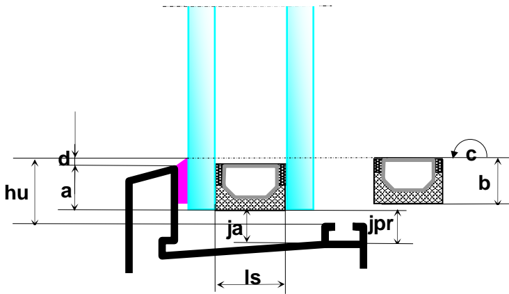
Détail en traverse basse
