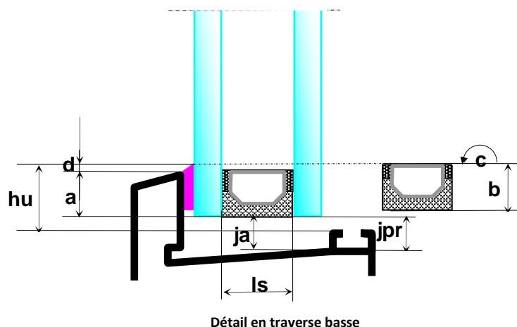
Détail en traverse basse
