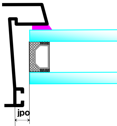
Détail en traverse haute et montants latéraux
